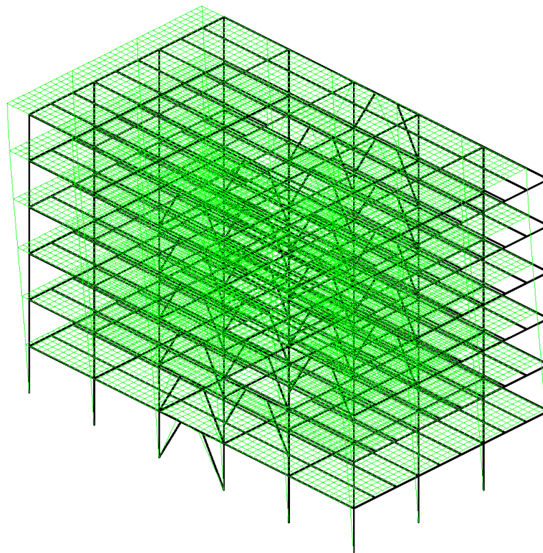
Izometrija Forma osciliranja: 2/10 [T=1.0484sec / f=0.95Hz]
