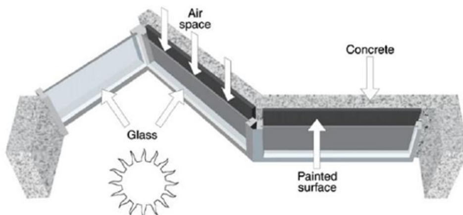
Slika 15. Cik-cak Trombeov zid
