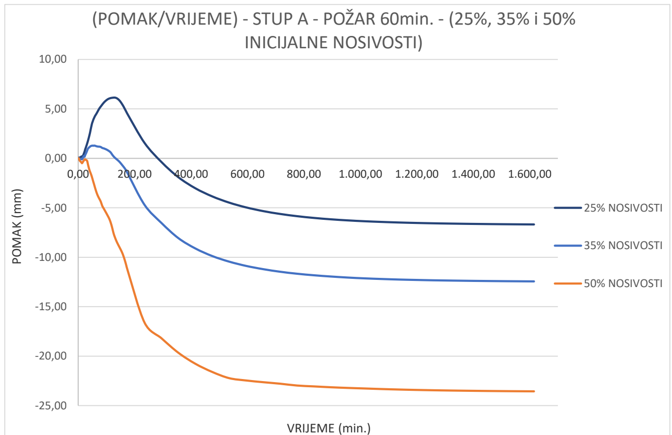
Slika 6.127: Prikaz dijagrama (pomak-vrijeme) za vrijeme požara od 60 minuta i različite intezitete opterećenja sile
