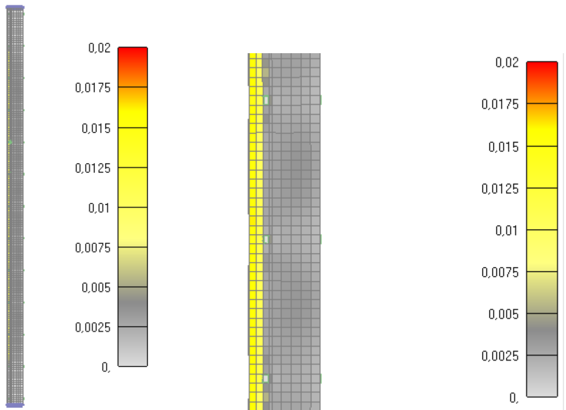
Slika 6.151: Prikaz pukotina za jednu četvrtinu stupa nakon 1030 minuta (lijevo-cijeli stup, desno-detalj stupa)
