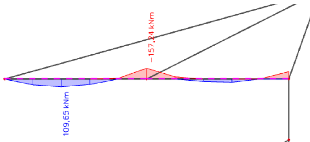
Prikaz vrijednosti momenta i položaja zatega kod rubnog nosača
