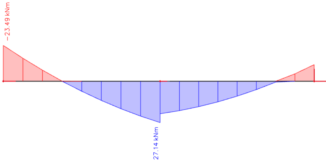
Slika 10.37 Maksimalni momenti savijanja M_y
