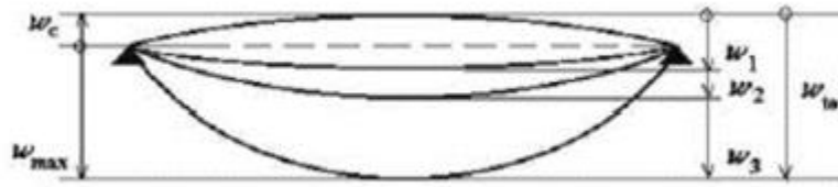
Slika 7.1.4 Prikaz progiba grede
