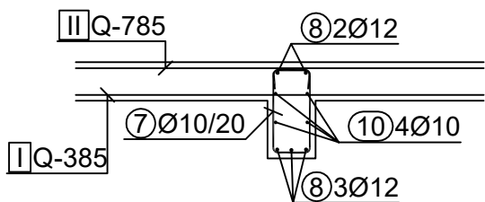
Presjek 2 - 2
