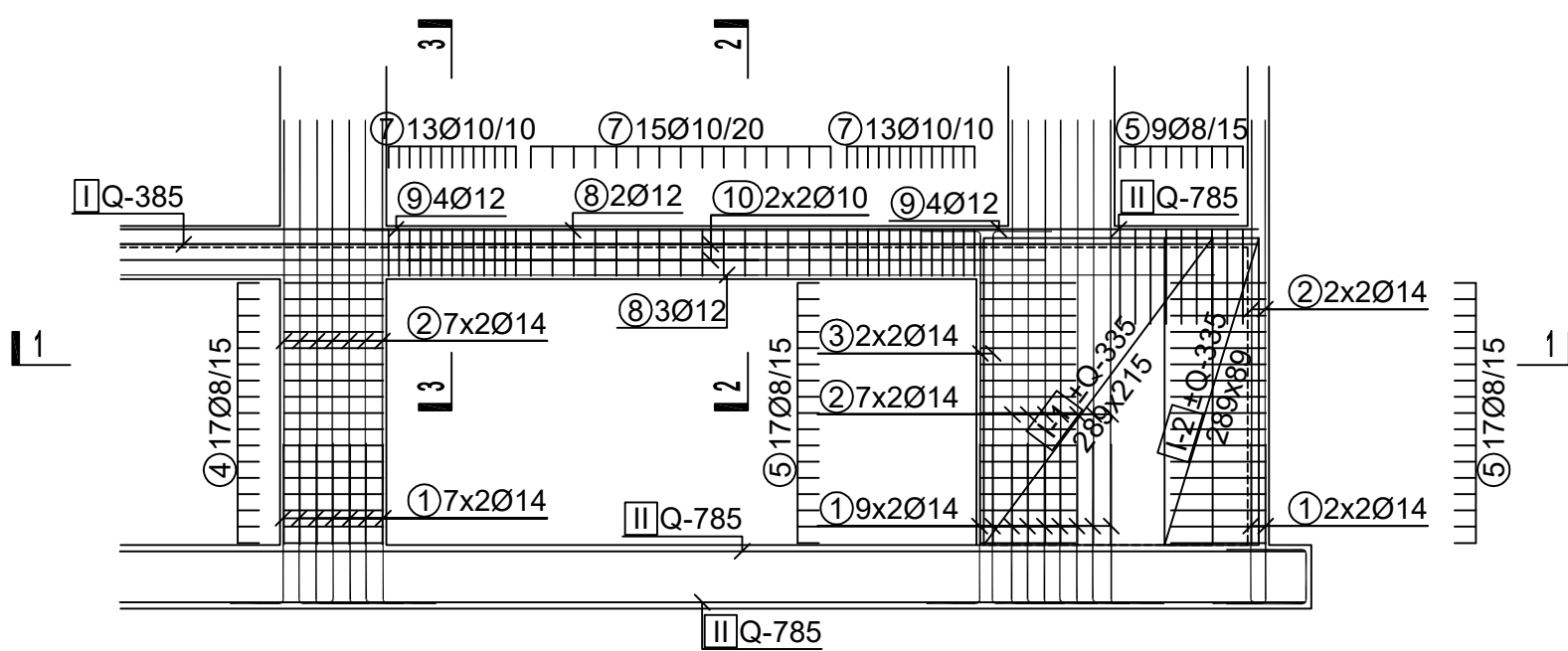
Presjek 1 - 1
