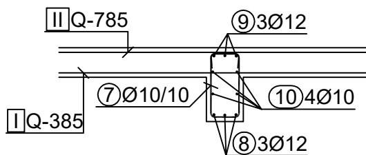
Presjek 3 - 3
