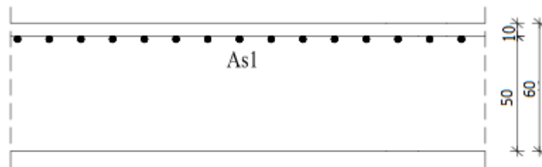
Slika 6.10. Skica armature u gornjoj zoni
