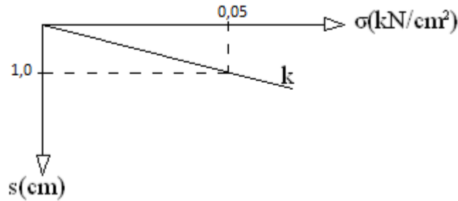
Slika 6.1. Dijagram odnosa napreznja u tlu i slijeganja
