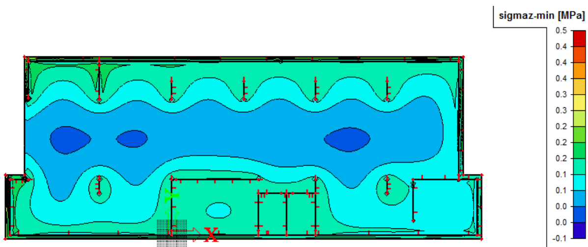
Slika 6.2.. Prikaz max. napreznja temeljne ploče
