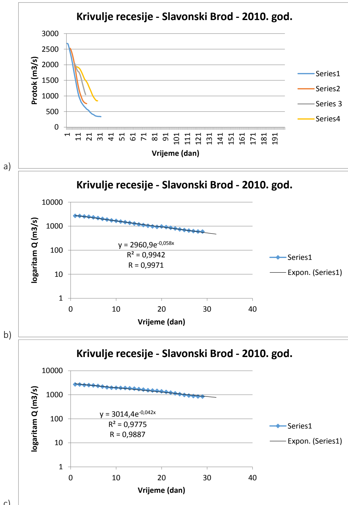
Slika 6.14.: Krivulje recesije – Slavonski Brod – 04.06.-19.10.2010. god. a) Izdvojene recesije, b) Krivulja pražnjenja „tabulation“ metodom, c) Krivulja pražnjenja „matching strip“ metodom
