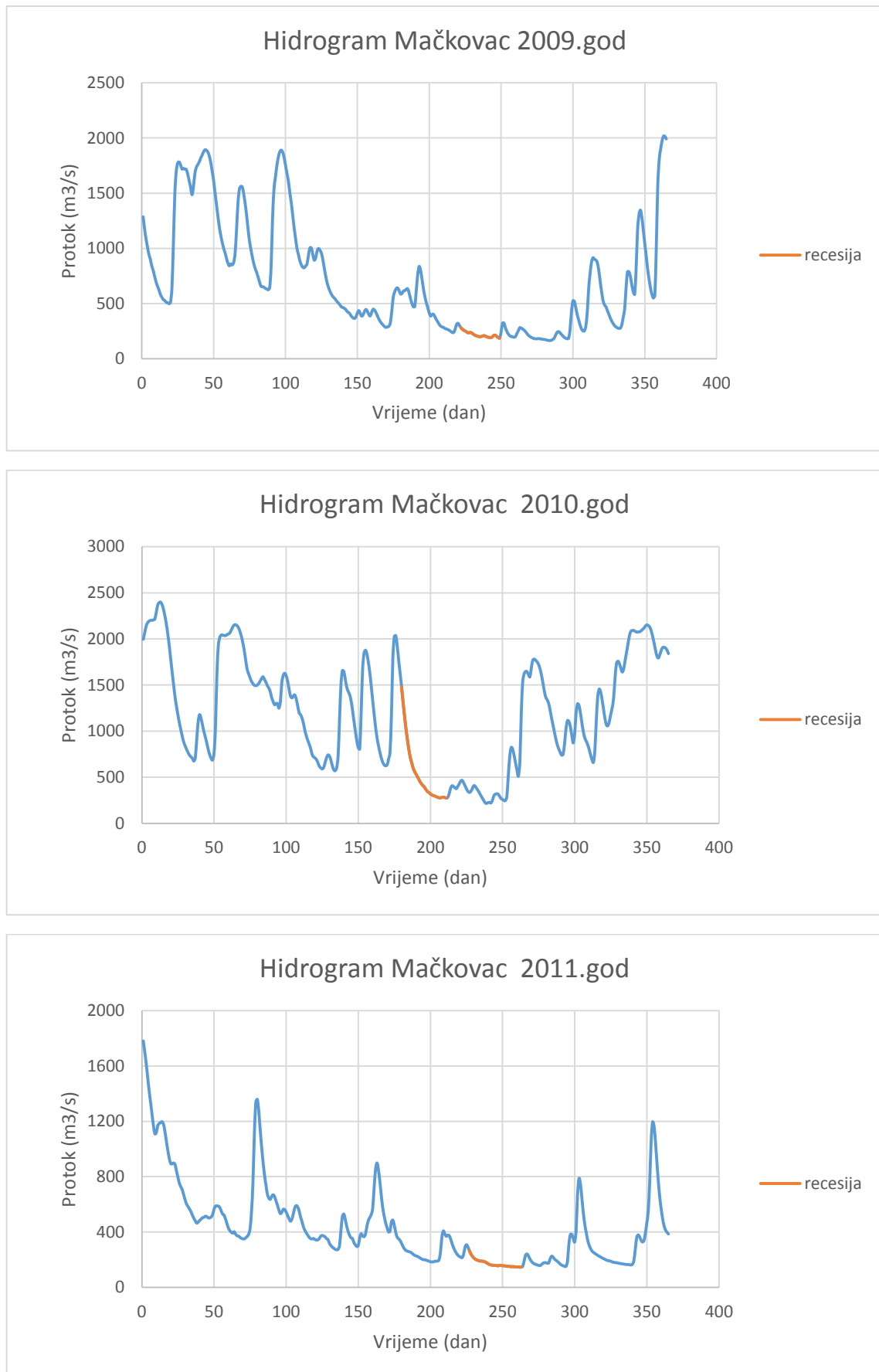
Slika 4.8.: Hidrografi za mjernu stanicu Mačkovac za 2009. – 2011. godinu
