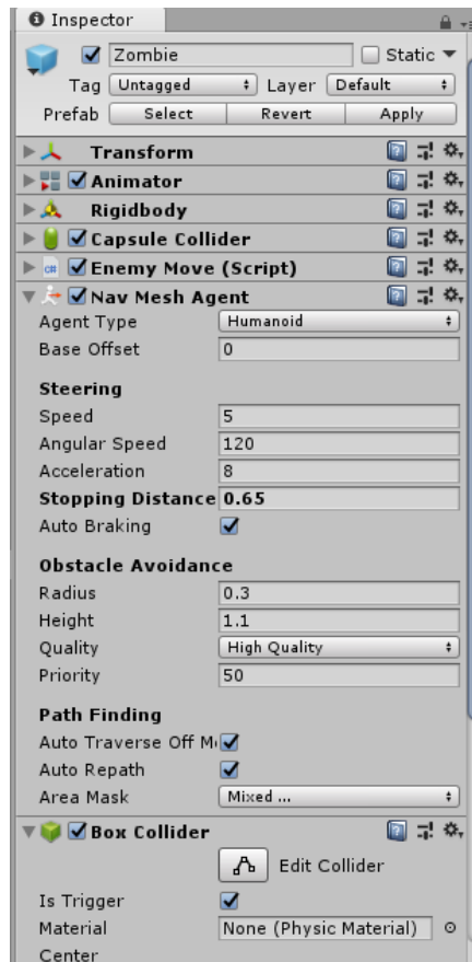
Slika 28. Nav Mesh Agent
