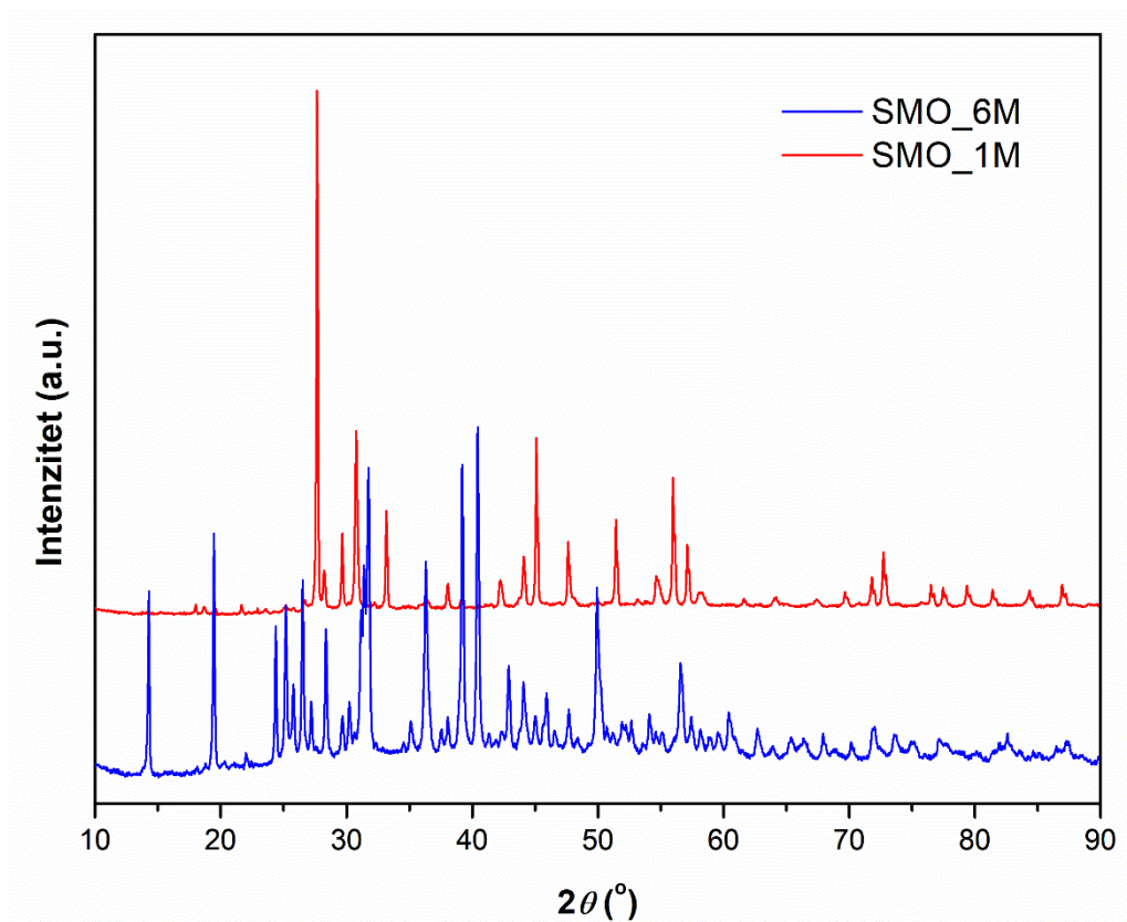
Slika 23. Difraktogrami uzoraka SMO_1M i SMO_6M.
