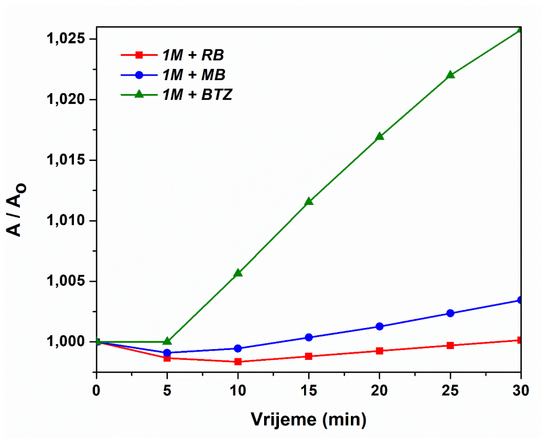
Slika 27. Ovisnost promjene apsorbancije ( A/A_0 ) o vremenu za interakciju SMO_1M fotokatalizatora sa rodaminom B, metilenom plavo i bromtiomolom zeleno.
