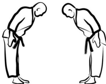
Slika 3. Judaški naklon
