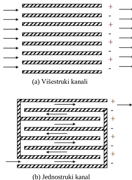
Slika 1.10. Načini protoka vode između elektroda. 13
