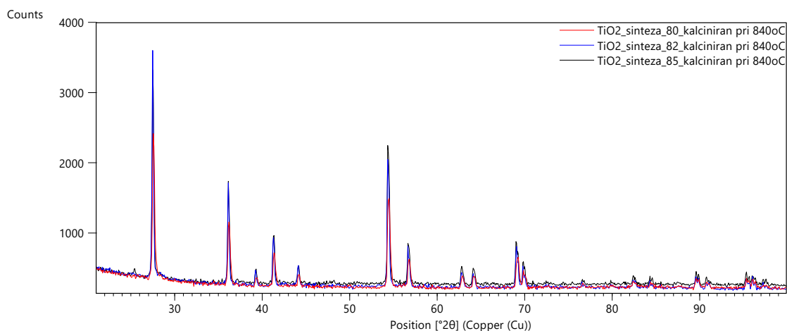
Slika 31. Difrakcijske slike uzorka TiO 2 nakon provedene kalcinacije u trajanju od 3 sata pri 840 °C
