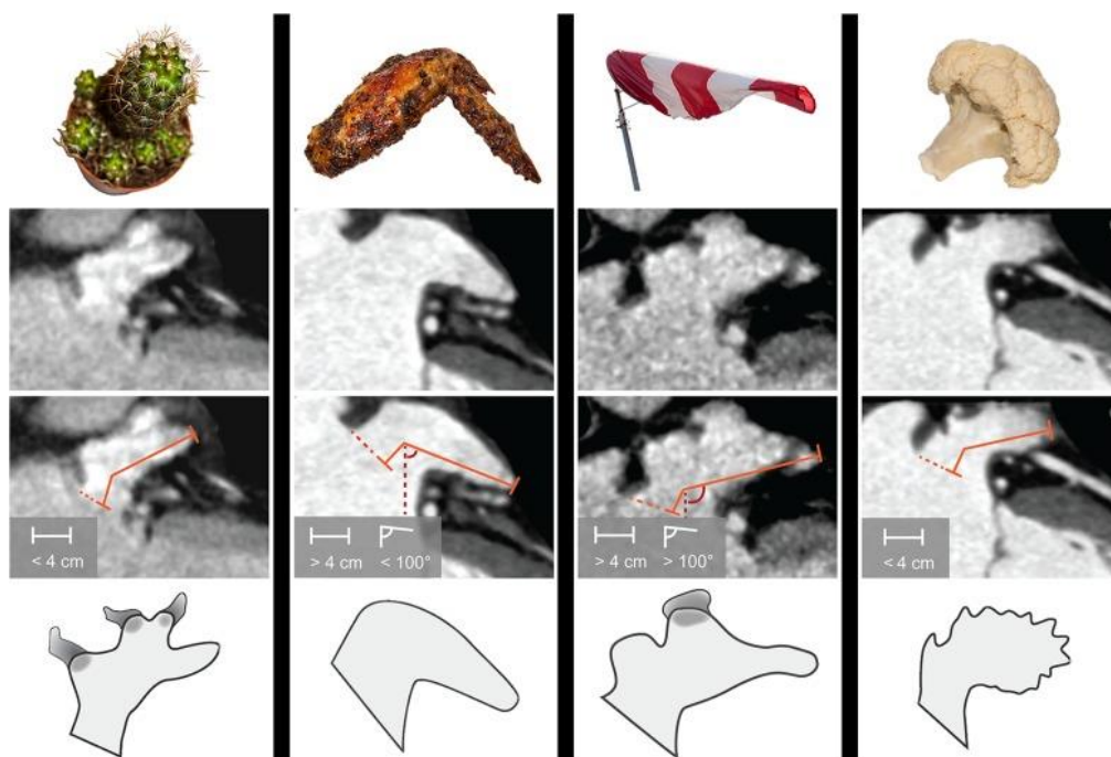
Slika 3. Morfološki oblici LAA. Oblik kaktusa ima jedan dominantan lobus s jednim ili više sekundarnih lobusa i duljinom manjom od 4 \text{ cm} . Oblik kokošnjeg krila ima samo jedan lobus duljine veće od 4 \text{ cm} s nagibom manjim od 100^\circ . Oblik vjetrulje ima jedan dominantan lobus s nekoliko sekundarnih i tercijarnih lobusa duljine veće od 4 \text{ cm} i nagibom većim od 100^\circ . Oblik cvjetače ima duljinu veću od 4 \text{ cm} s kompleksnom unutarnjom strukturom. 8
