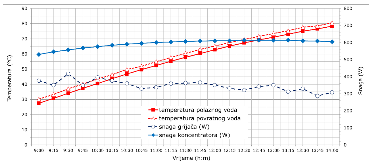
Slika 4.5. – Snaga solarnog paraboličnog koncentrataora i promjena temperature vode pri odvodu i dovodu u spremnik
