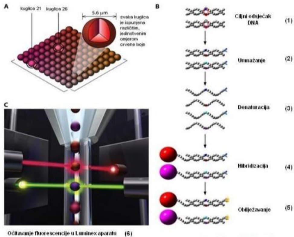
Slika 18. Proces hibridizacije
