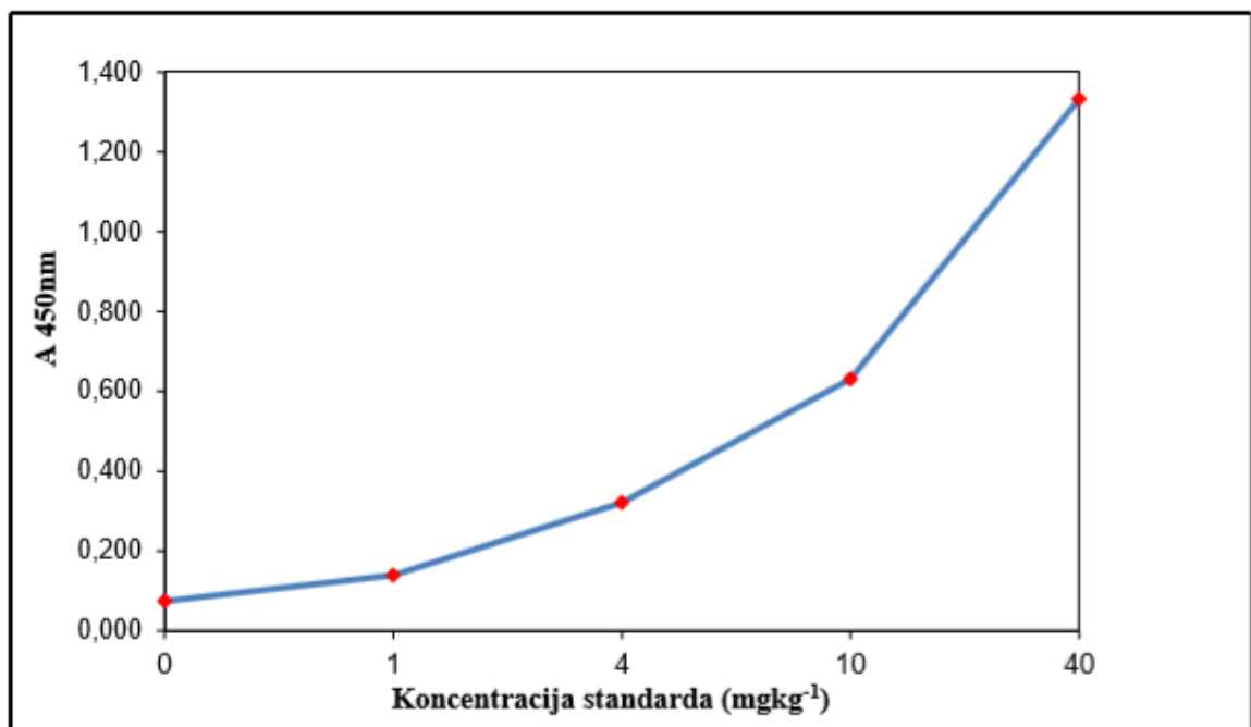
Slika 10. Baždarni dijagram standarda kikirikija
