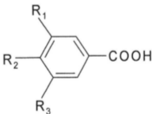
Slika 7. Struktura hidroksibenzojeve kiseline (Robards i sur., 1999)
