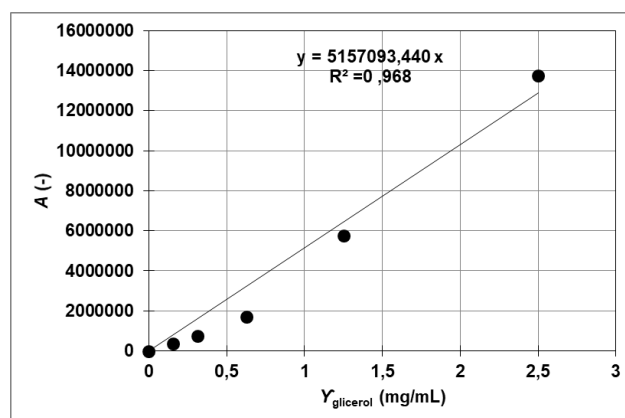
Slika 5. Baždarni dijagram za određivanje koncentracije glicerola
