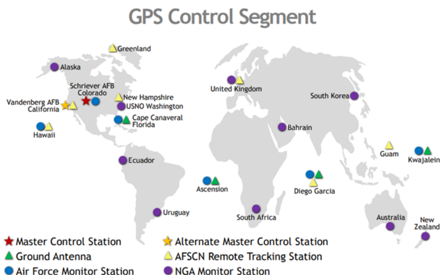
Slika 16. Kontrolni segment GPS-a Izvor: https://www.gps.gov/systems/gps/space/
