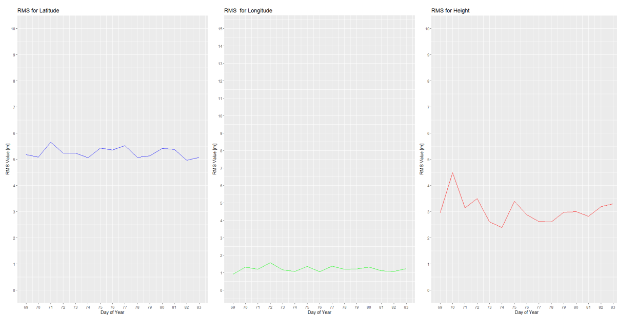
Slika 39. Vrijednosti srednje kvadratne pogreške za stanicu THU s modelom ispravke (ON) Izvor: Izradio autor obradom podataka u programu Rstudio
