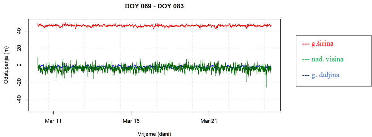
Slika 41. Modelirane vrijednosti odstupanja položaja za period od 10. do 24. ožujka 2015. (NYAL) Izvor: Izradio autor obradom podataka u programu Rstudio
