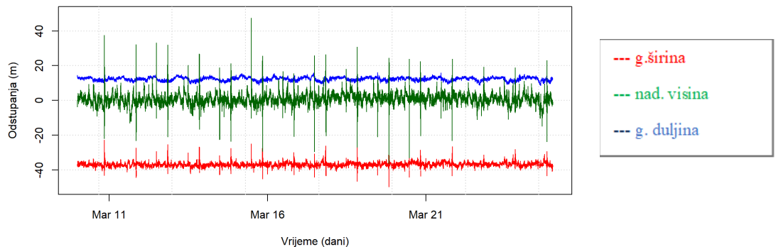
Slika 49. Odstupanja modeliranih vrijednosti za period od 10. do 24. ožujka 2015. godinu (SCORE) Izvor: Izradio autor obradom podataka u programu Rstudio
