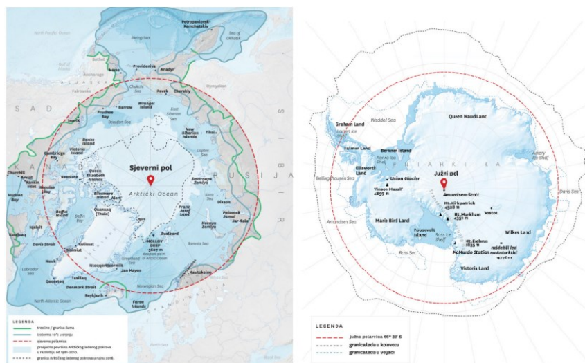
Slika 1. Područja Sjevernog pola (lijevo) i Južnog pola (desno)
