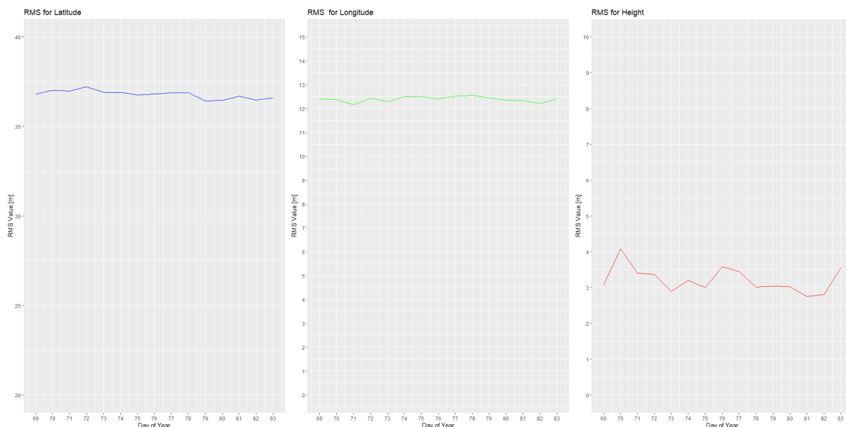
Slika 55. Vrijednosti srednje kvadratne pogreške za stanicu SCOR s modelom ispravke (ON) Izvor: Izradio autor obradom podataka u programu Rstudio
