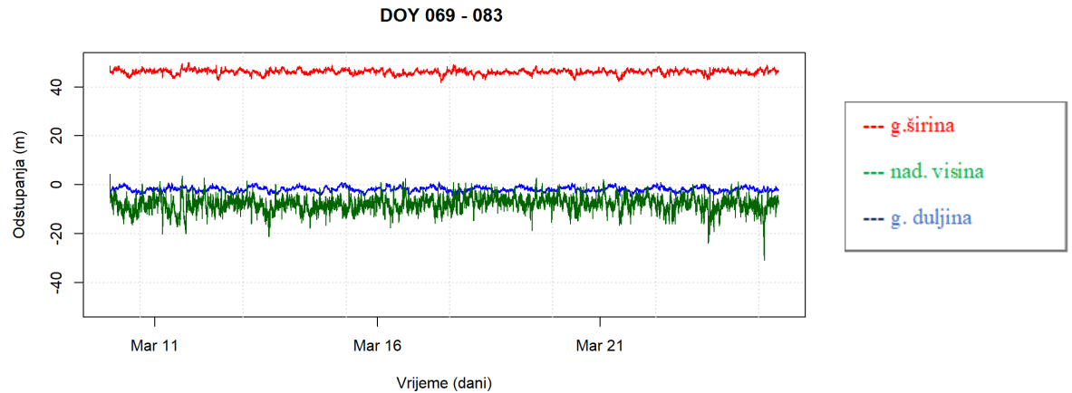
Slika 40 Nemodelirane vrijednosti odstupanja položaja za period od 10. do 24. ožujka 2015. (NYAL) Izvor: Izradio autor obradom podataka u programu Rstudio
