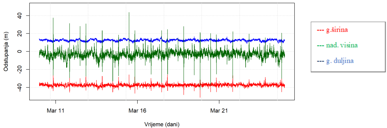
Slika 48. Odstupanja za nemodelirane vrijednosti u periodu od 10. do 24. ožujka 2015. godine (SCORE) Izvor: Izradio autor obradom podataka u programu Rstudio
