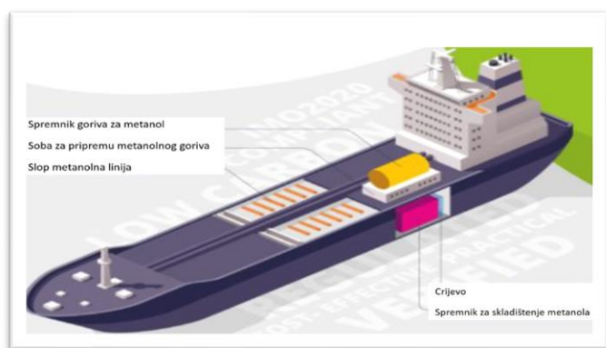
Slika 6: Prikaz izgleda broda koji koristi metanol [6]
