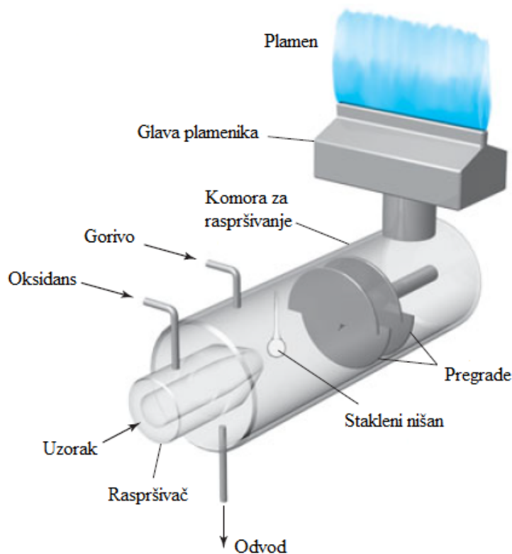
Slika 2. Plameni atomizator laminarnog protoka (preuzeto i prilagođeno prema: Harris, 2010)
