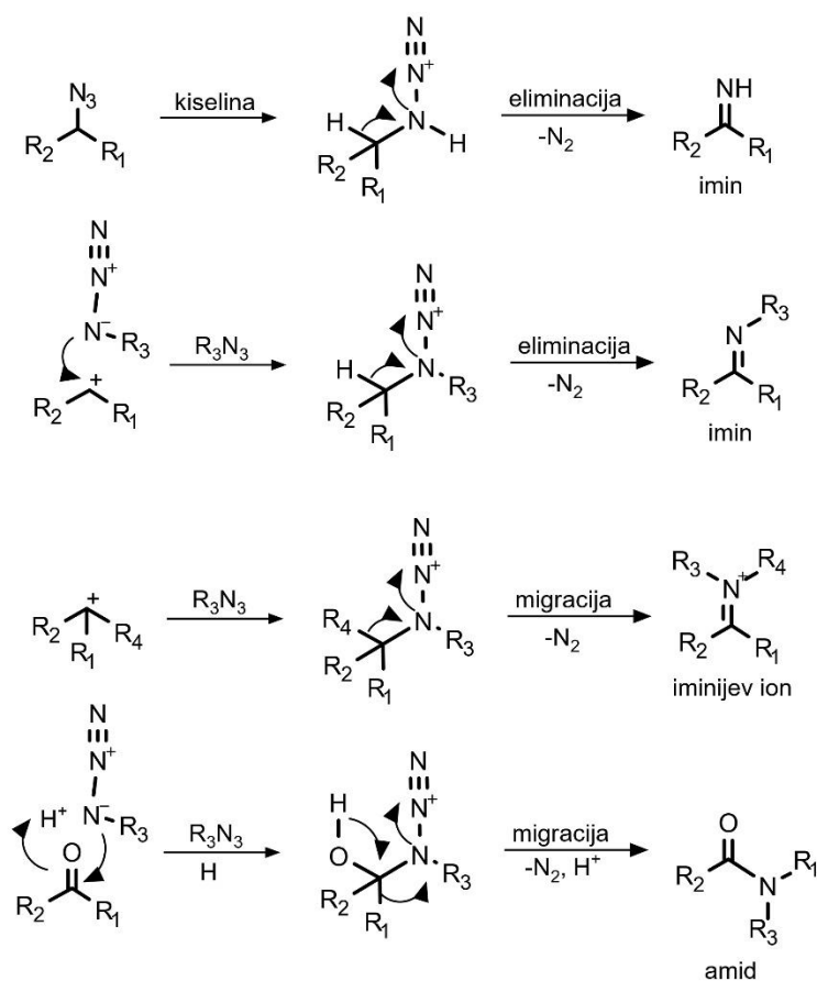
Shema 2. Prikaz Schmidtove reakcije preraspodjele
