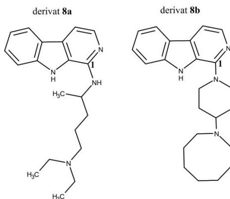
Slika 19. 1-amino- \beta -karbolinski derivati
