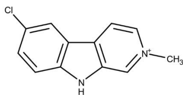
Slika 2. Strukturna formula nostokarbolina
