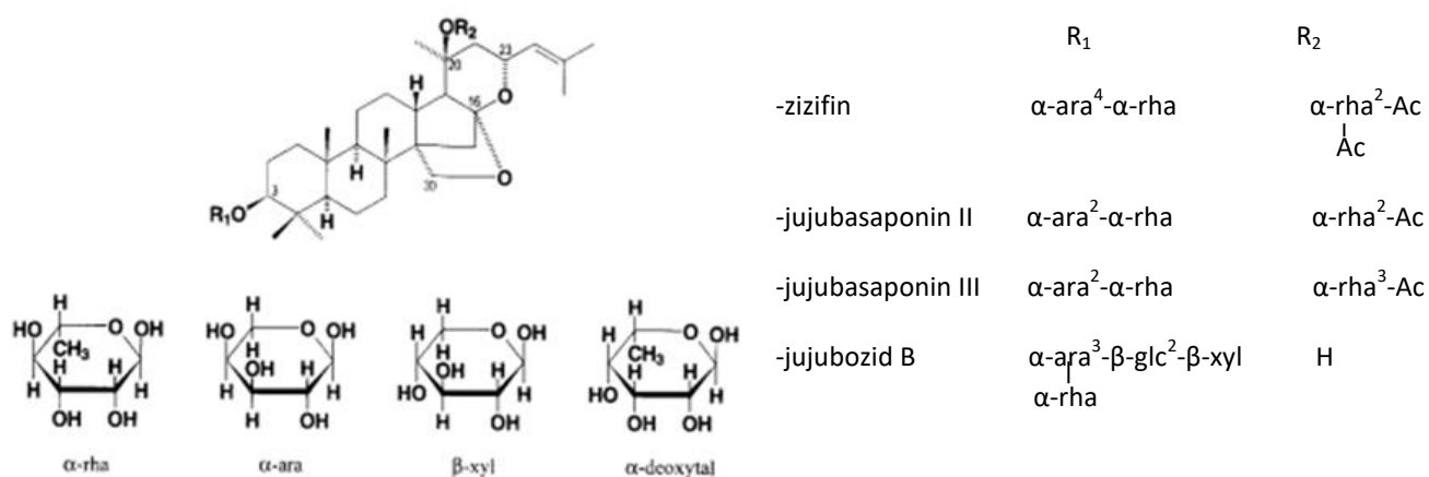
Slika 7. Kemijske strukture nekih saponina (Suttisri i sur., 1995)
