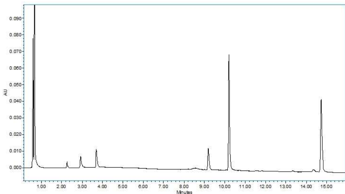
Slika 10: Kromatogram odjeljivanja aktivne sastavnice i onečišćenja s dihidrogenfosfatnim puferom kao mobilnom fazom (vrijeme gradijenta 30 min, temperatura kolone 40°C).
