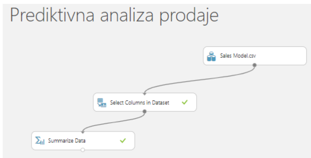
Slika 4.9. Dijagram modela nakon statističke obrade podataka
