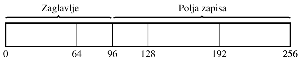
Slika 2.1: Horizontalni zapis
