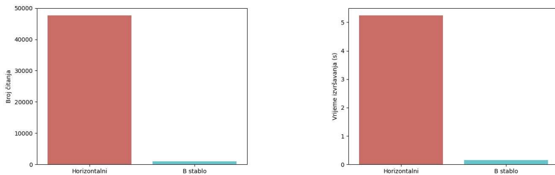
Slika 5.2: Pretraživanje raspona
