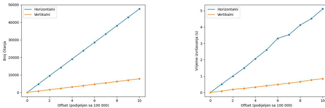
Slika 3.5: Dohvat zapisa po primarnom ključu
