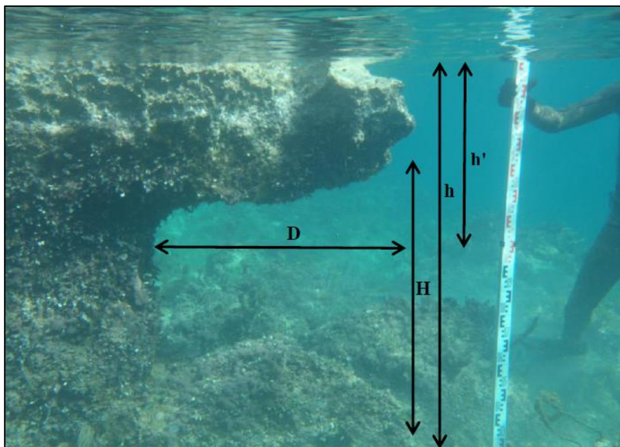
Sl. 9. Profil plimne potkapine br. 18 (lokacija 3); prikaz mjerenih geometrijskih parametara
