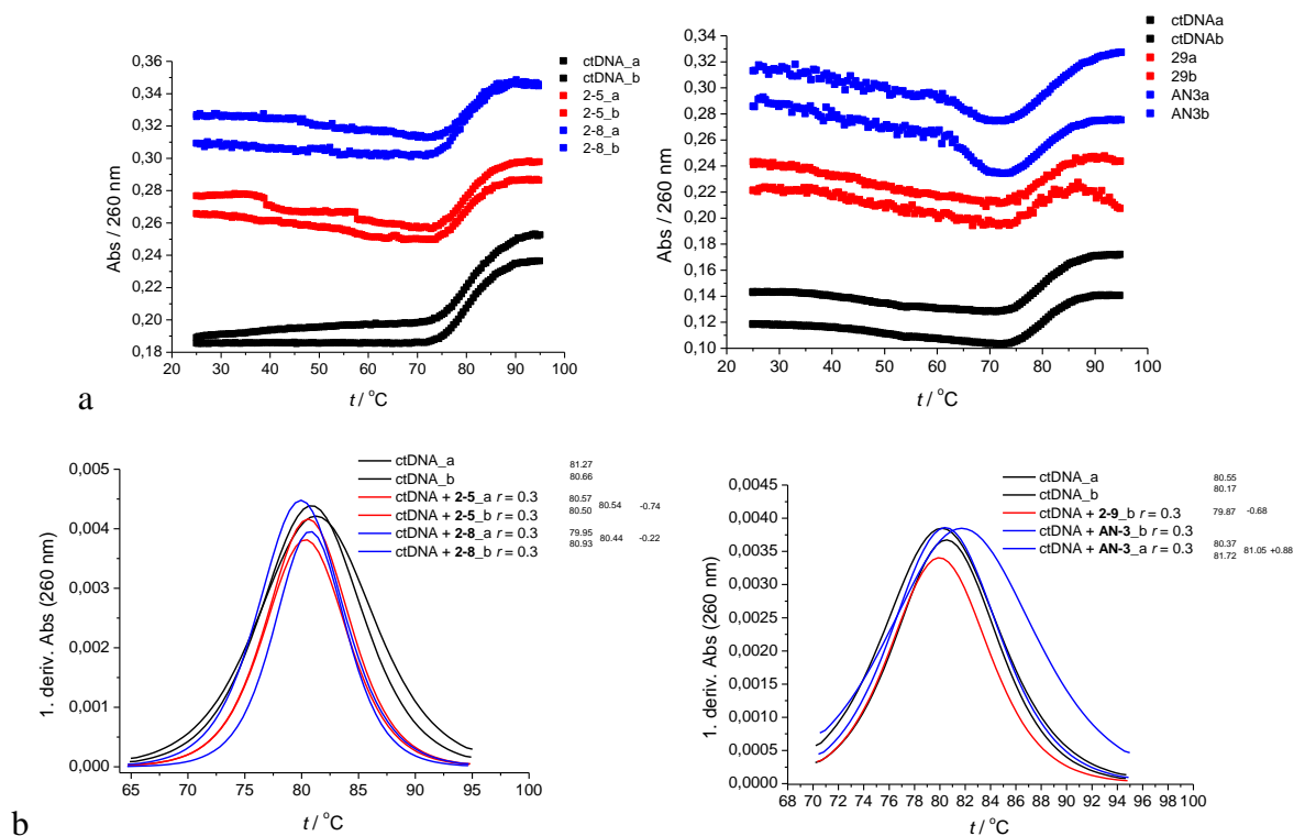
Slika D24. a) krivulja mekšanja ct -DNA uz dodatak spojeva 2-5 , 2-8 , 2-9 i AN-3 u omjeru r_{\text{[spoj]}/[\text{polinukleotid}]} = 0,3 u Na-kakodilatnom puferu ( I = 0,05 \text{ mol dm}^{-3} , pH= 7,0) i b) prva derivacija denuracijske krivulje ct -DNA
