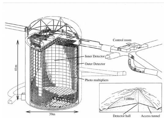
(b) Shematski prikaz Super-Kamiokande detektora.
