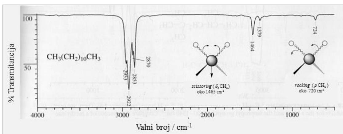
Slika 2.3.3.1. Prikaz asigniranog IR spektra dodekana sa pripadajućim vibracijama: C-H istežanja: simetrično ( 2870\text{ cm}^{-1} ) i asimetrično ( 2953\text{ cm}^{-1} ) \text{CH}_3 , simetrično ( 2853\text{ cm}^{-1} ) i asimetrično ( 2922\text{ cm}^{-1} ) \text{CH}_2 , C-H savijanja: simetrično \text{CH}_2 ( 1464\text{ cm}^{-1} ), simetrično ( 1379\text{ cm}^{-1} ) i asimetrično ( 1450\text{ cm}^{-1} ) \text{CH}_3 , ljuljanje \text{CH}_2 ( 724\text{ cm}^{-1} ) 10
