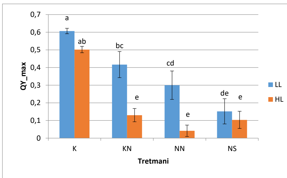
Slika 8 Maksimalni kvantni prinos fotosustava II (QYmax) za uzorke Evernia prunastri mjereno 7. dana nakon tretmana. Tretmani: K – kontrola, lišajevi prskani vodom pH vrijednosti 6,5, KN – lišajevi tretirani otopinom kalijeva nitrata ( c=1 M, pH=6,5 ), NN – lišajevi tretirani otopinom amonijeva nitrata ( c=1 M, pH=6,5 ), NS – lišajevi tretirani otopinom amonijeva sulfata ( c=0,5 M, pH=6,5 ), HL- svjetlo jačeg intenziteta ( 100 \mu E m^{-2} s^{-1} ), LL – svjetlo slabijeg intenziteta ( 40 \mu E m^{-2} s^{-1} ). Različita slova iznad stupaca predstavljaju statistički značajno različite rezultate ( p < 0,05 ).
