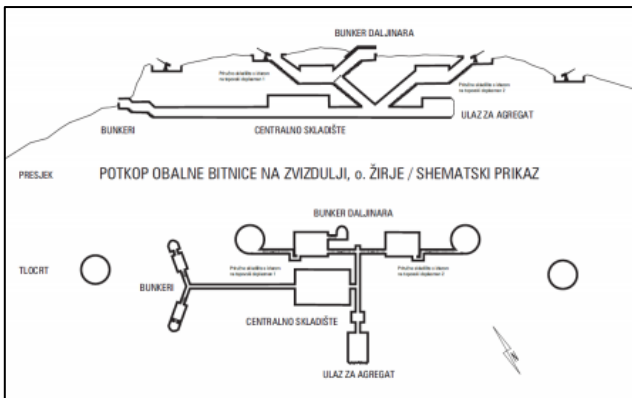
Sl. 11. Shema potkopa na Žirju
