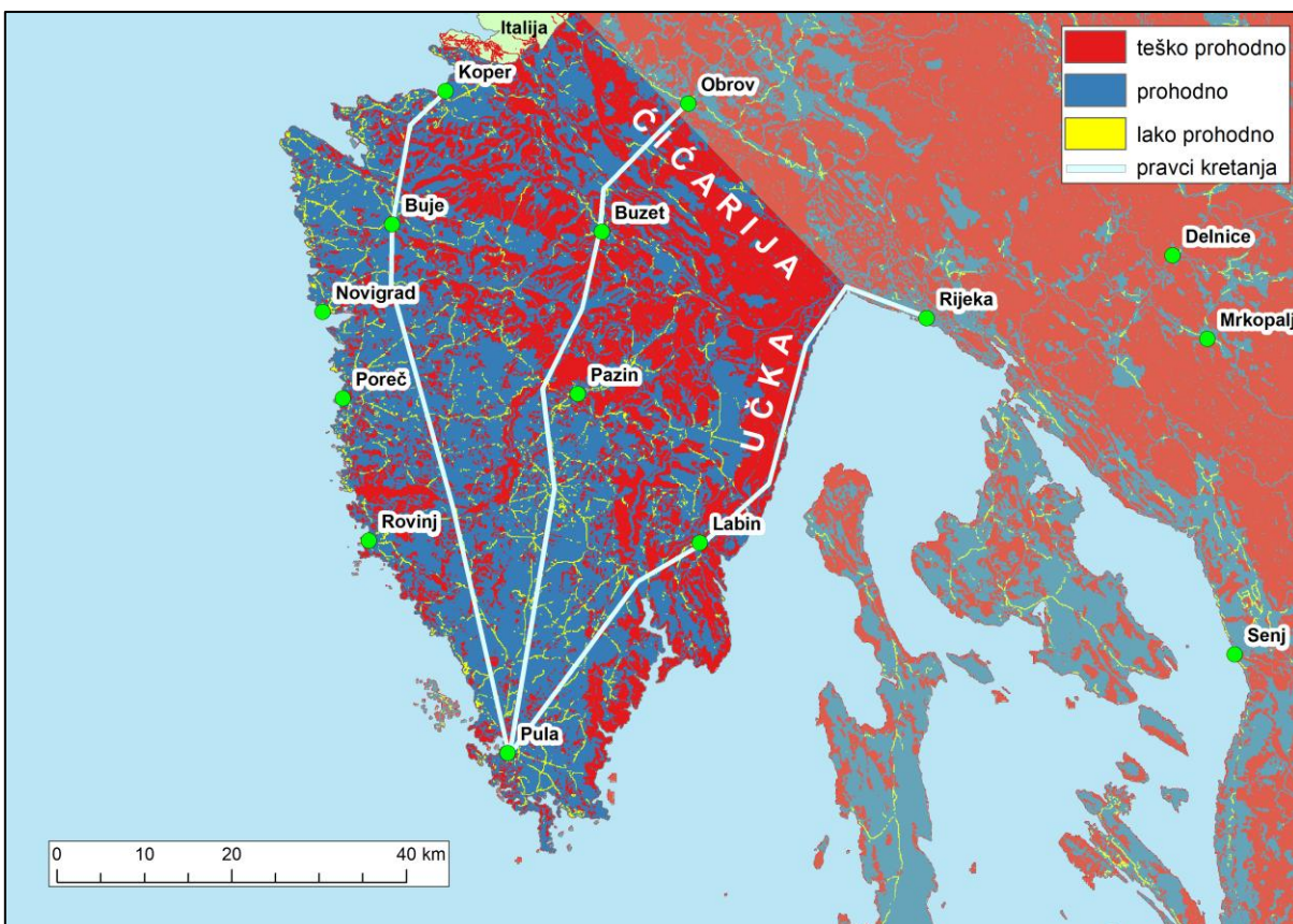
Sl. 28. Prohodnost istarske pomorsko-desantne osnovice
