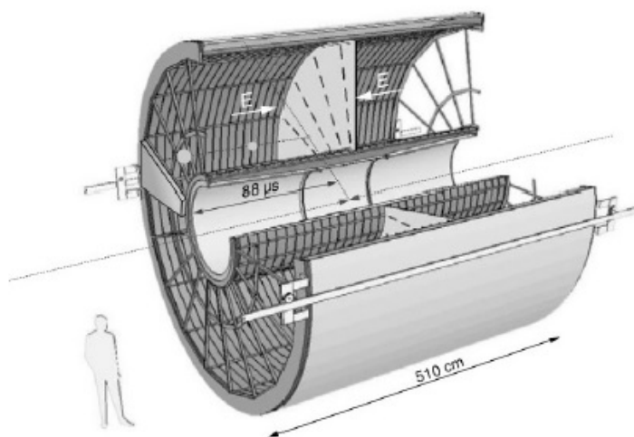
Slika 3.4: Shema TPC-a
