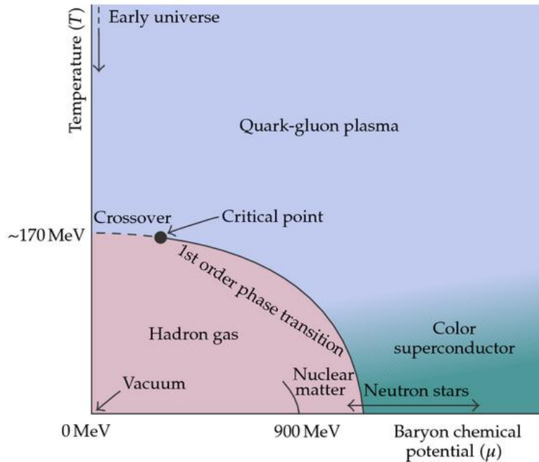
Slika 2.2: Fazni dijagram
