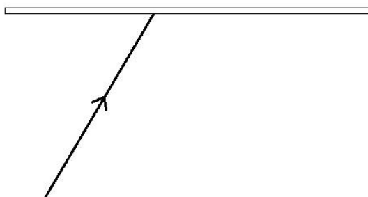
Slika 6.1. Zraka svjetlosti upada na ravno zrcalo.
