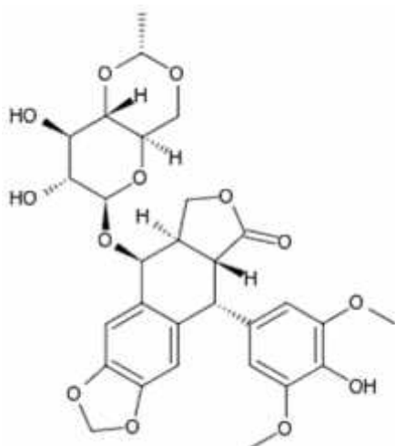
Slika 9. Molekula etopozida
