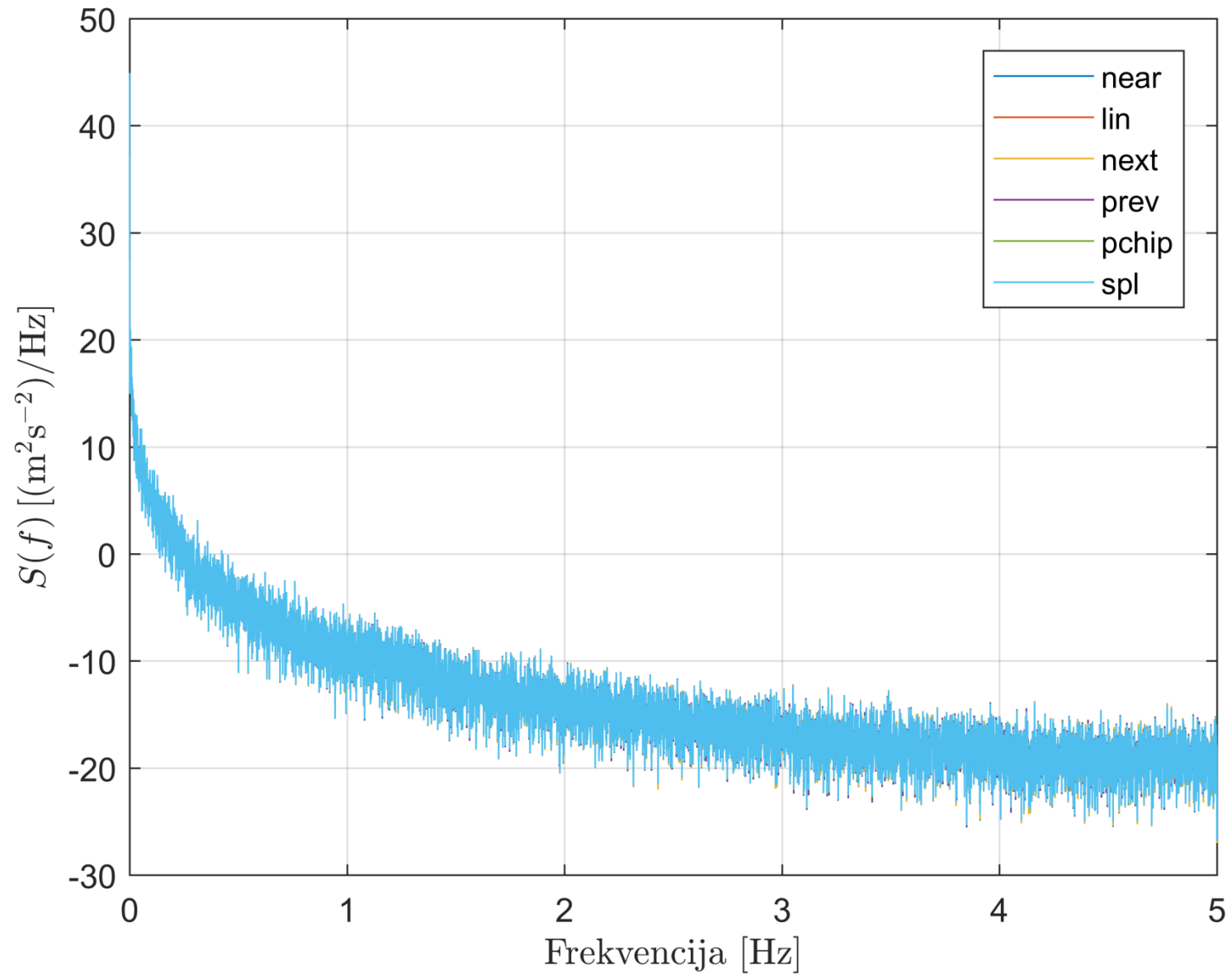
Slika 3.3: Spektralna gustoća snage u komponente "bure 1a" (tablica 2.1) na visini 10 m s vrstama interpolacije kao na slici 3.2. Razlike u spektru između interpolacija su zanemarive (omjer reda veličine razlika i reda veličine spektra je 0,01).
