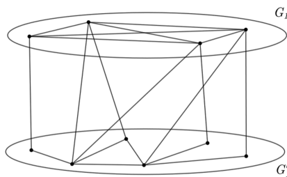
Slika 2.5: Graf G
