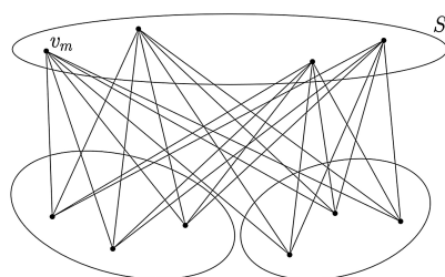
Slika 2.8: Turanov graf
