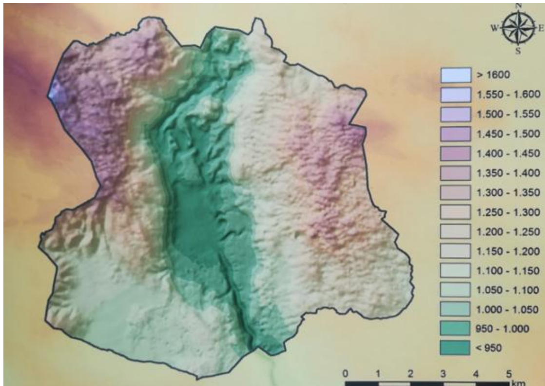
Sl. 7 Hipsometrijska karta područja Šujice (Radoš, 2014)
