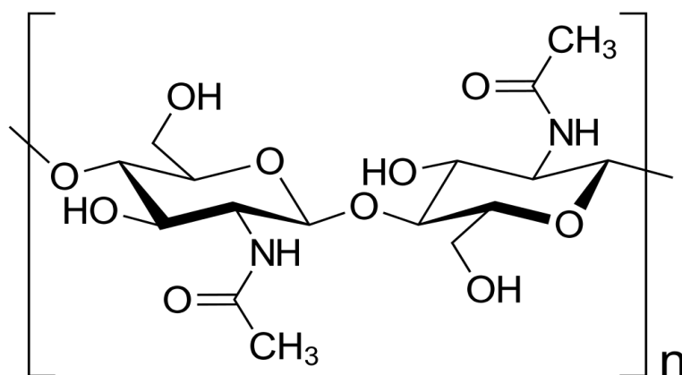
Slika 11. Struktura hitina
