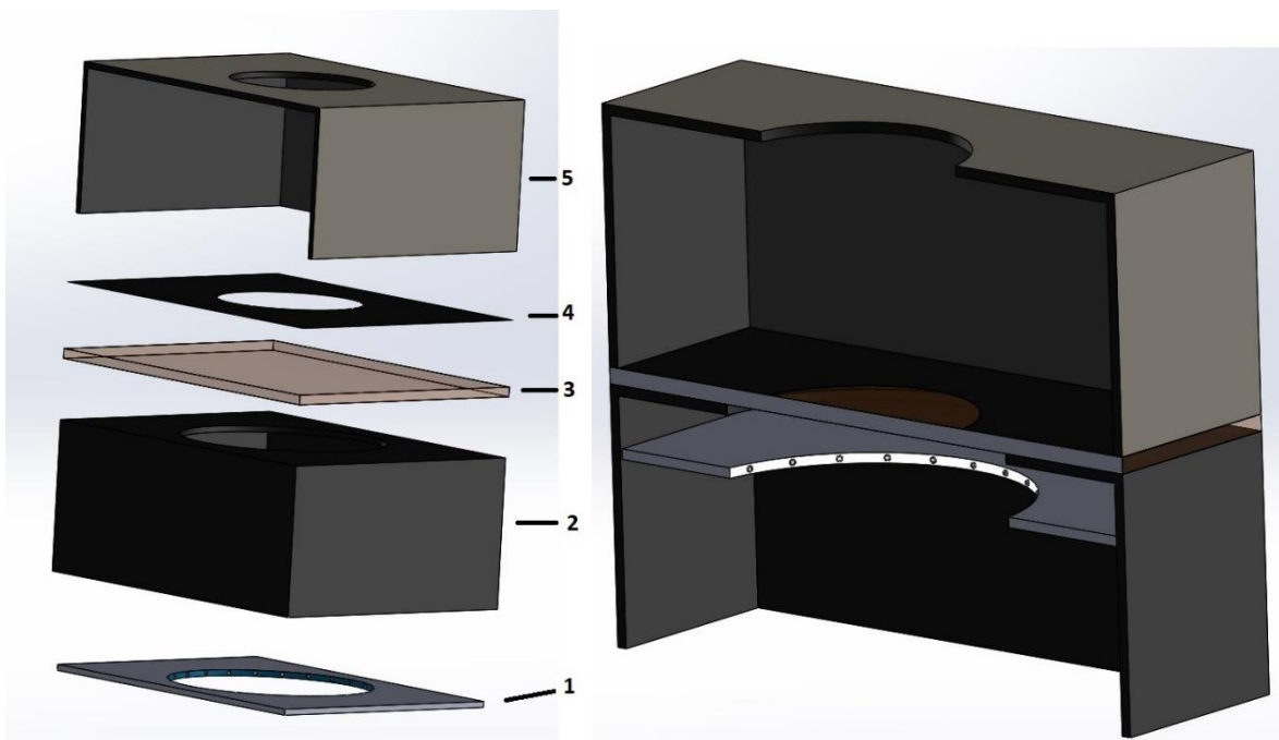
Slika 4 Redoslijed sklapanja povećala (lijevo), poprečni presjek povećala (desno)
