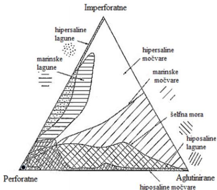
Slika 13 Prikaz trokomponentnog dijagrama za određivanje okoliša s obzirom na tip stijenki za uzorak K2 (modificirano prema Murray, 1974)
