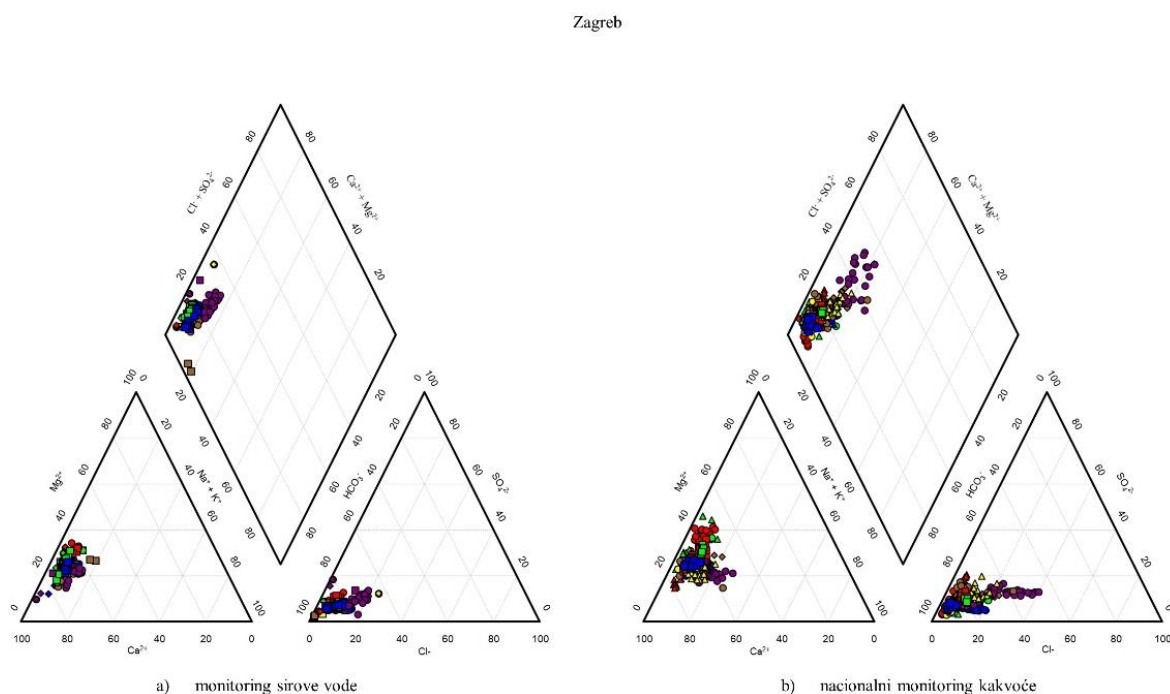
Slika 7-12. Piperovi dijagrami GTPV-a Zagreb
