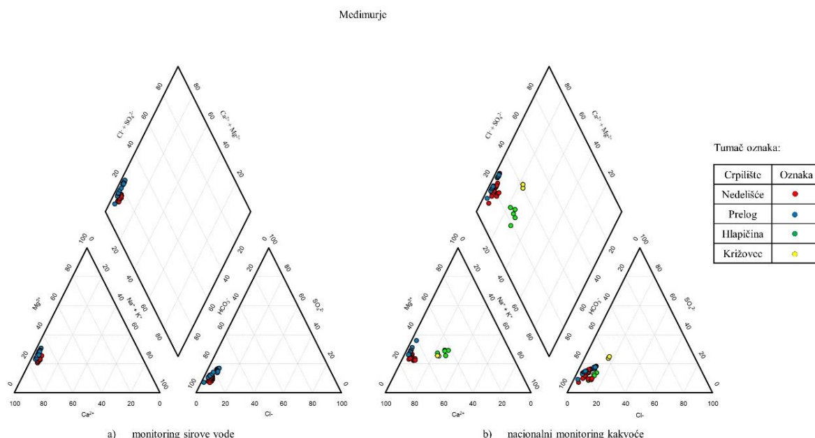
Slika 7-1. Piperovi dijagrami GTPV-a Međimurje
