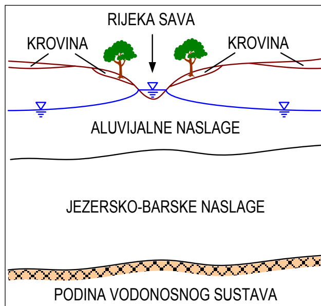
Slika 2.4. Shematski profil samoborsko-zaprešićkog vodonosnika (preuzeto iz Posavec, 2006).
