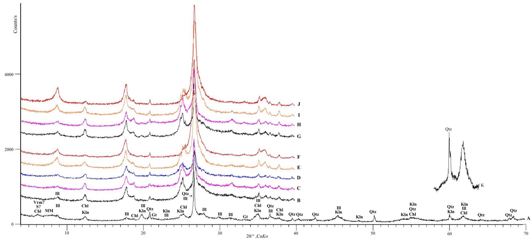
Slika 5-31. Difrakcijske slike glinovite frakcije uzorka 4896 (A i K predstavljaju snimke neorijetiranih uzorkaka, a B – J snimke orijetiranih uzoraka): A - netretirani uzorak, B - uzorak tretiran s K^+ , C - uzorak tretiran s K^+ saturiran s etilen-glikolom, D - uzorak tretiran s K^+ saturiran s dimetilsulfoksidom, E - uzorak tretiran s K^+ žaren na 350^\circ C , F - uzorak tretiran s K^+ žaren na 550^\circ C , G - uzorak tretiran s Mg^{2+} , H - uzorak tretiran s Mg^{2+} saturiran s etilen-glikolom, I - uzorak tretiran s Mg^{2+} žaren na 350^\circ C , J - uzorak tretiran s Mg^{2+} žaren na 550^\circ C ; K - difrakcijska linija 060. Tumač kratica: Qtz – kvarc, Chl – klorit, Ill – illitični materijal, Gt – getit, Kln – kaolinit, MM-miješanoslojni minerali glina, Vrm – vermikulit, S – smektit.
