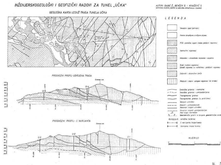
Slika 3-3. Inženjersko-geološka karta s pripadajućim profilima.
