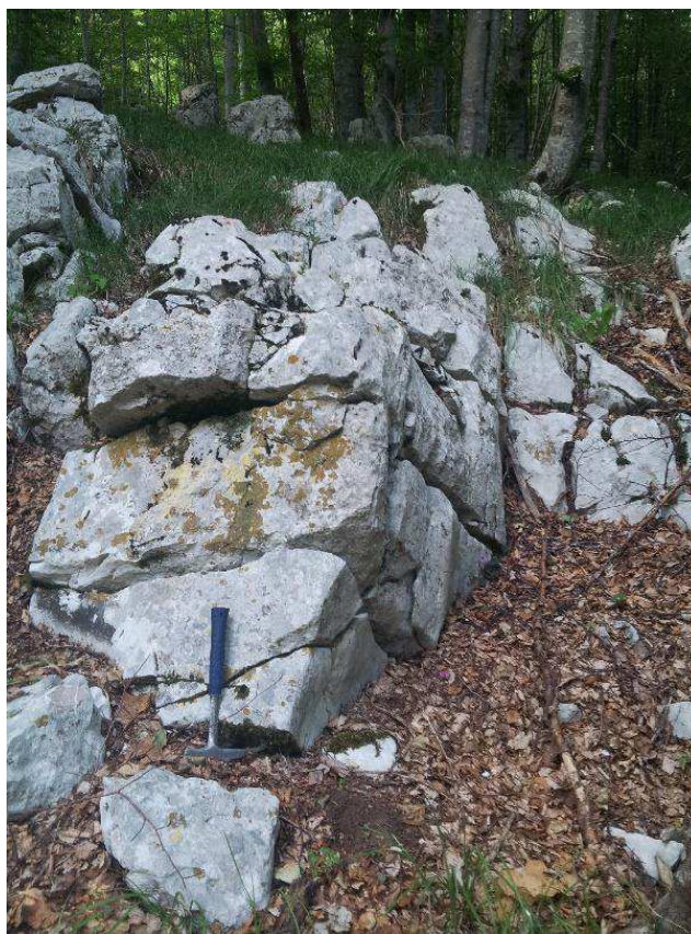
Slika 5-19. Slojeviti izdanak foraminiferskog vapnenca na točki D 135 .
