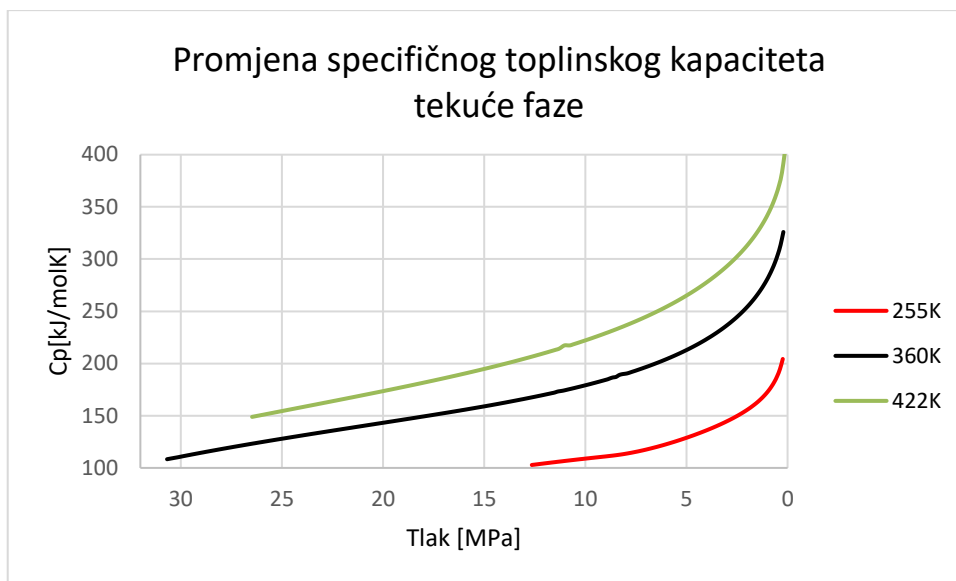
Slika 4-8. Rezultati proračuna specifičnog toplinskog kapaciteta tekuće faze
