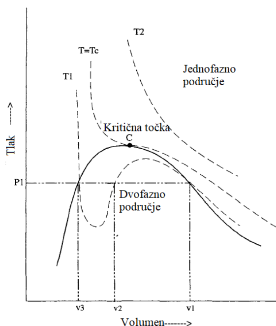
Slika 2-6. Volumetrijsko ponašanje ležišnog fluida izračunato van der Waalsovom kubičnom jednačbom stanja (van der Waals, 1873)
