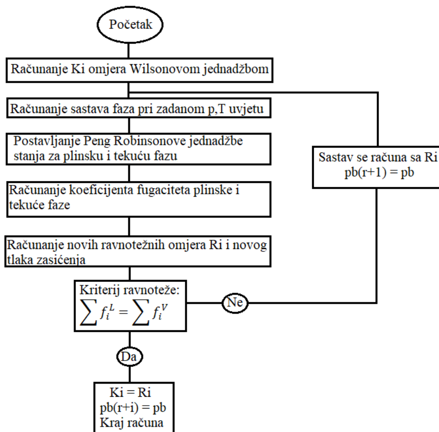
Slika 3-1. Procedura računanja fazne ravnoteže kubičnom jednačbom stanja
