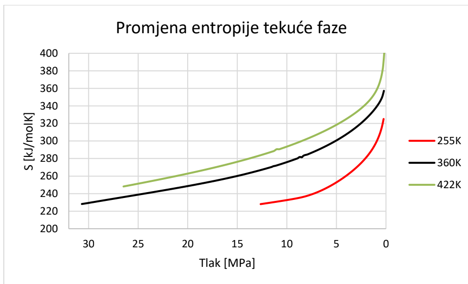
Slika 4-6. Rezultati proračuna entropije tekuće faze
