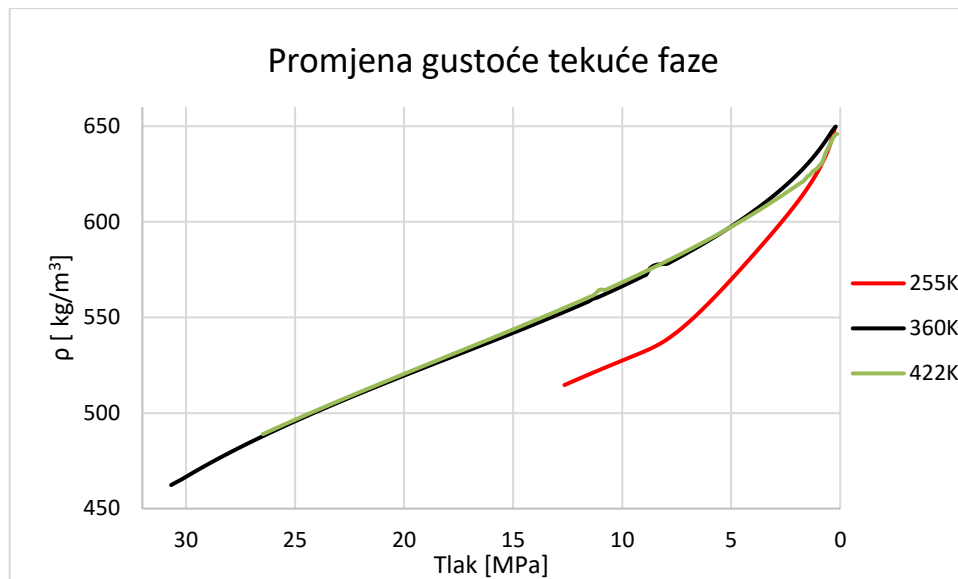
Slika 4-4. Rezultati proračuna gustoće tekuće faze
