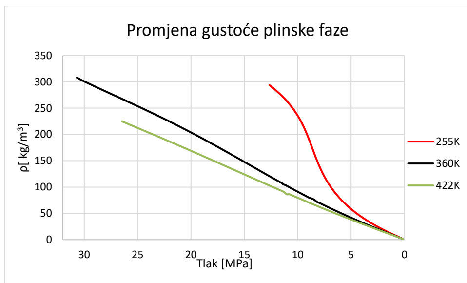
Slika 4-5. Rezultati proračuna gustoće plinske faze
