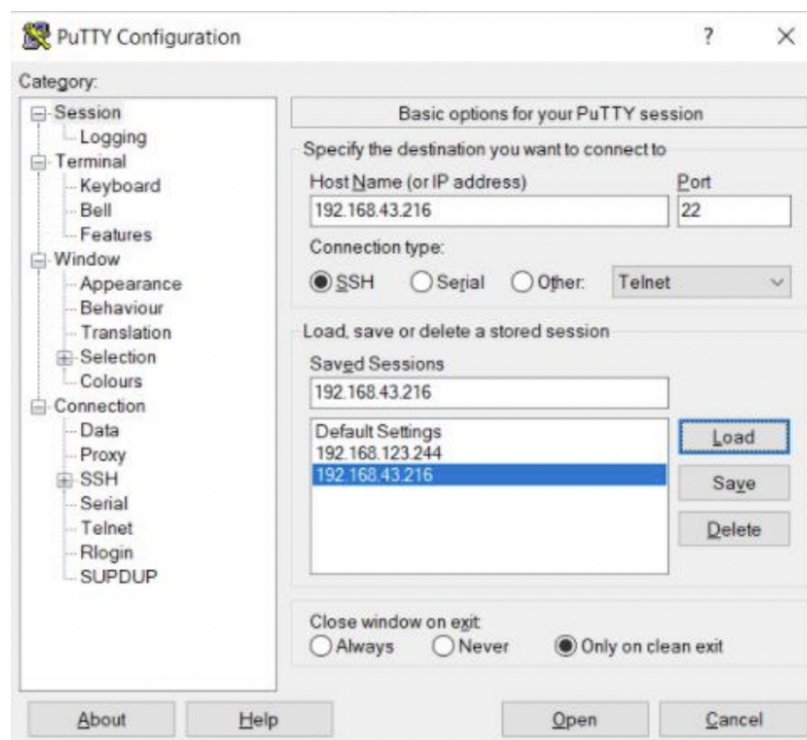
Slika 3.3.1 PuTTY konfiguracija
