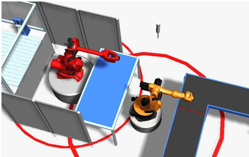
Slika 5.46 Verzija s kolaborativnim robotom - kobotom
