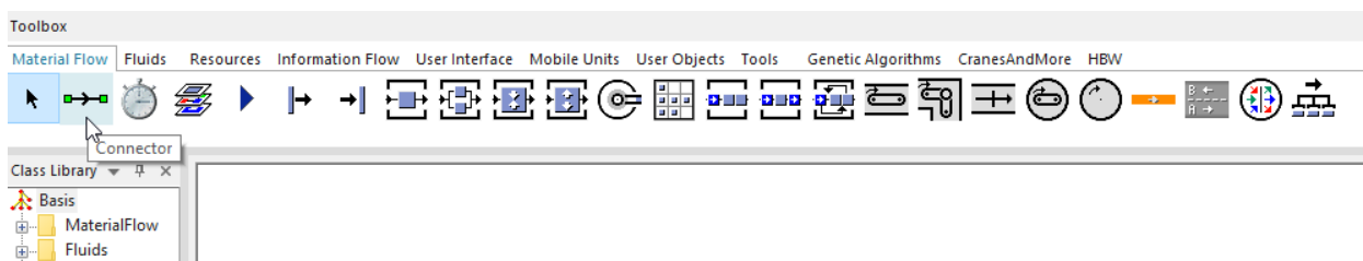
Slika 5.26 Objekt -Connector
