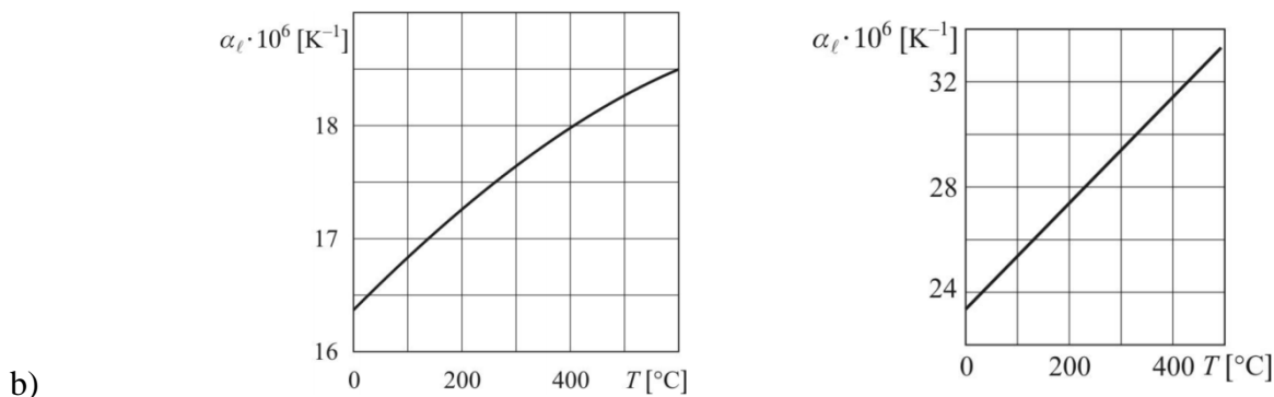
Slika 4. Utjecaj temperature na svojstva bakra i aluminija [17]:
